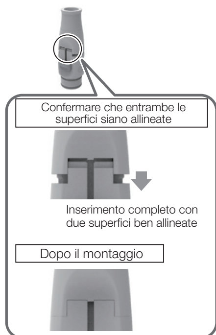
Manipolo di aspirazione
