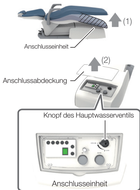
Knopf des Hauptwasserventils
