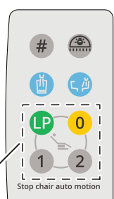
Helferinnen-Bedienfeld (Ausführung mit Helferinneneinheit)
