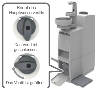
S3/S4 Ständer
